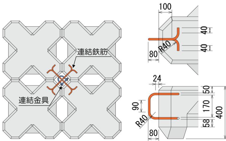
図-4.ラティス0.5t型の連結鉄筋と連結方法
