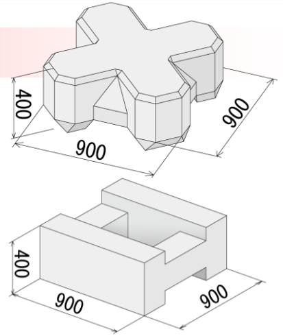
図-1.ラティスと標準平型
