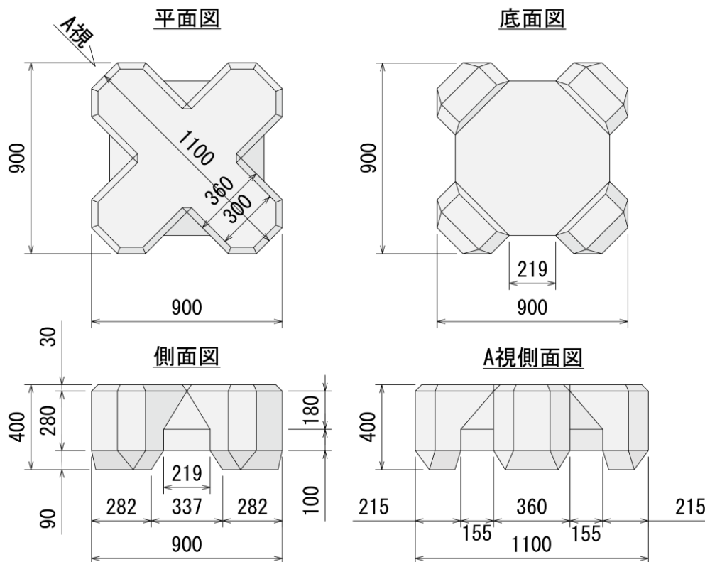
図-2.ラティス 0.5t 型 形状図
