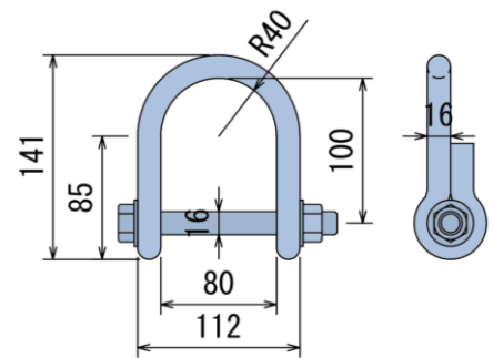
図-5.連結金具（φ16）
