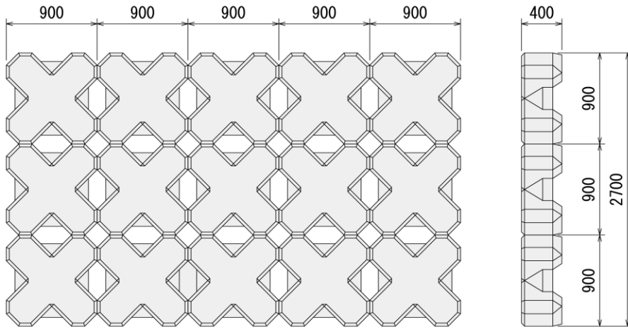
図-3.ラティス0.5t型の標準配列
